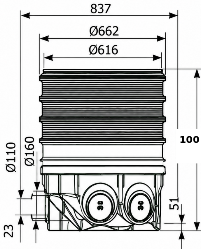
שוחה מוזרקת קוטר 60 גובה 100
