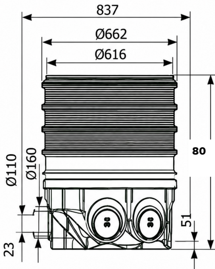
שוחה מוזרקת קוטר 60 גובה 80
