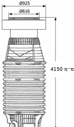
תא בקרה ECO100 קוטר 100 בסיס 5 כניסות קוטר 200 גובה 415 ס"מ
