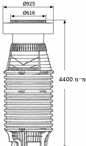
תא בקרה ECO100 קוטר 100 בסיס 5 כניסות קוטר 200 גובה 440 ס"מ
