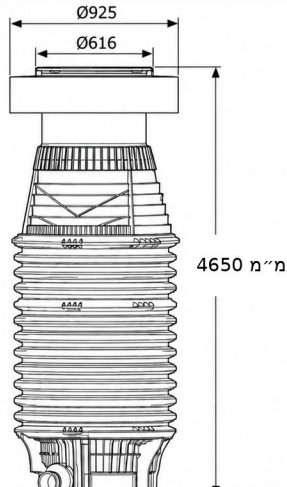
תא בקרה ECO100 קוטר 100 בסיס 5 כניסות קוטר 200 גובה 465 ס"מ
