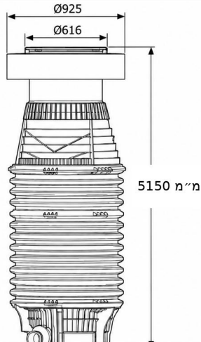
תא בקרה ECO100 קוטר 100 בסיס 5 כניסות קוטר 200 גובה 515 ס"מ
