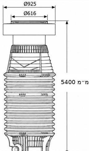
תא בקרה ECO100 קוטר 100 בסיס 5 כניסות קוטר 200 גובה 540 ס"מ
