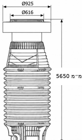
תא בקרה ECO100 קוטר 100 בסיס 5 כניסות קוטר 200 גובה 565 ס"מ
